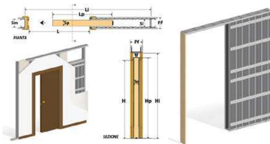
פרט לכיס גבס
