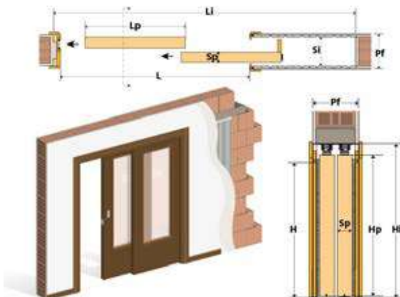
פרט לכיס בודד עם שתי דלתות נגררות
