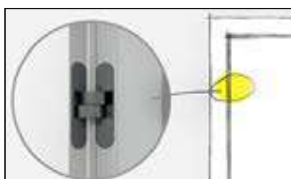
צירי SOS נסתרים
