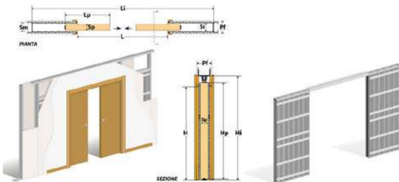
כיס גבס 2 דלתות
