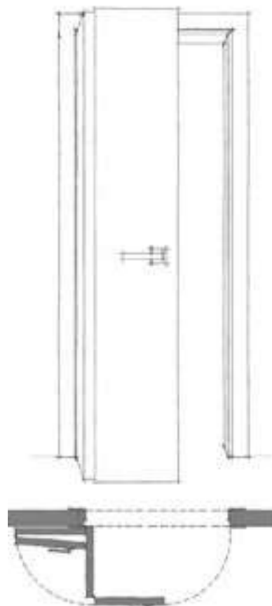
דלת הזזה מתקפלת
