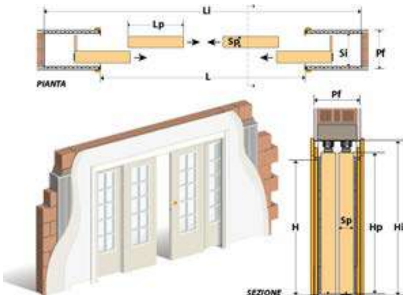
כיס כפול לפתח כפול - ארבע דלתות
