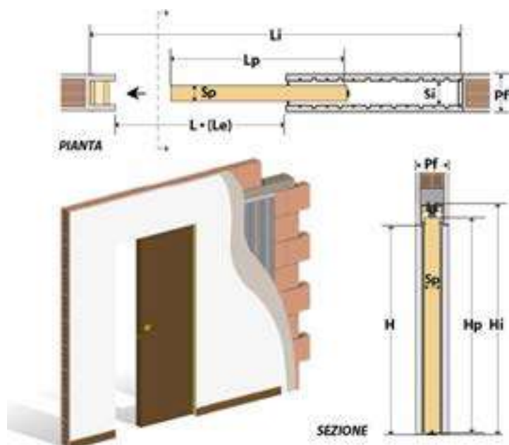
פרט לכיס בקו אפס ללא הלבשות
